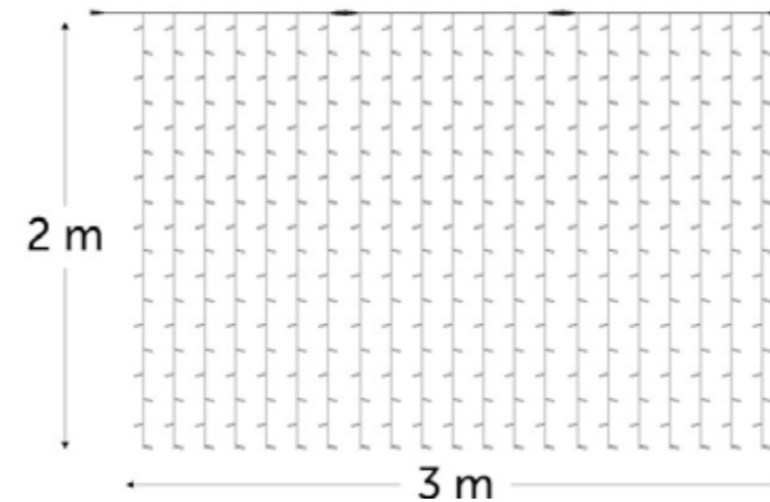
Droplight fixe ou flash Dimension : 300x200cm 378 led blanc chaud - IP44 - 24V
